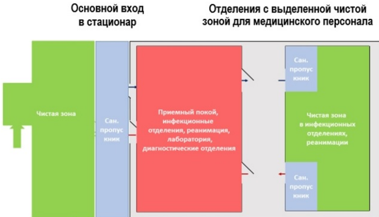
Схема модульного инфекционного стационара
